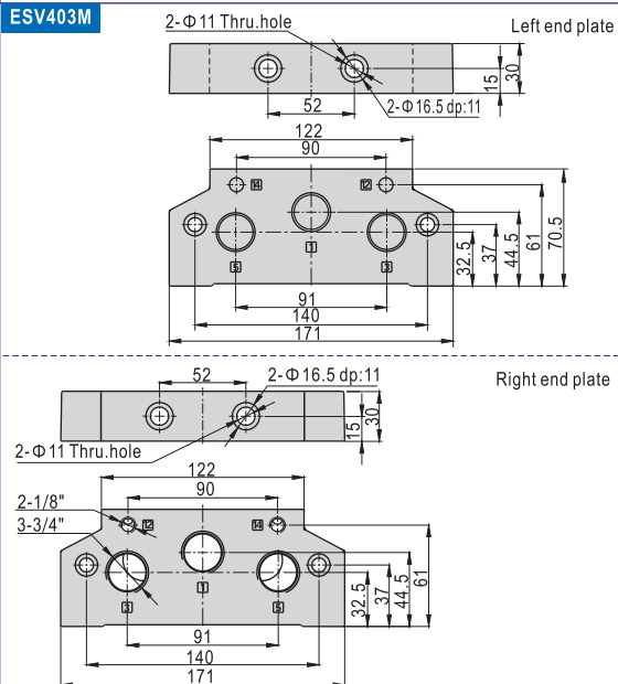
ESV403M
