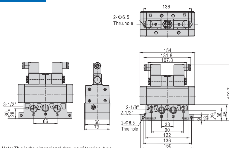
ESV430+ESV401M
