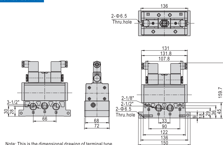
ESV420+ESV401M
