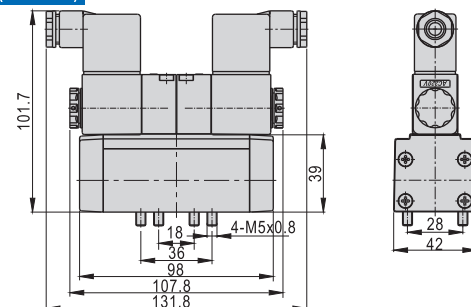
ESV230C(EIP) (Grommet)
