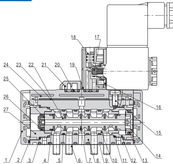
ESV210 (Terminal)
