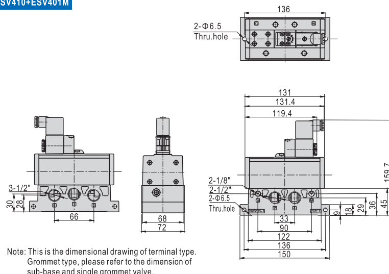
ESV410+ESV401M
