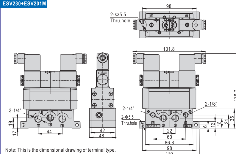
ESV230+ESV201M
