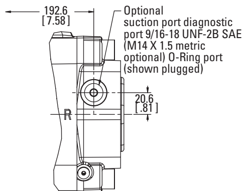
View A-A
